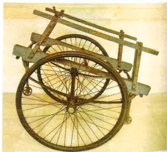
L'ingénieuse poussette porte-brancard Peugeot. The ingenious Peugeot stroller stretcher-carrier.
